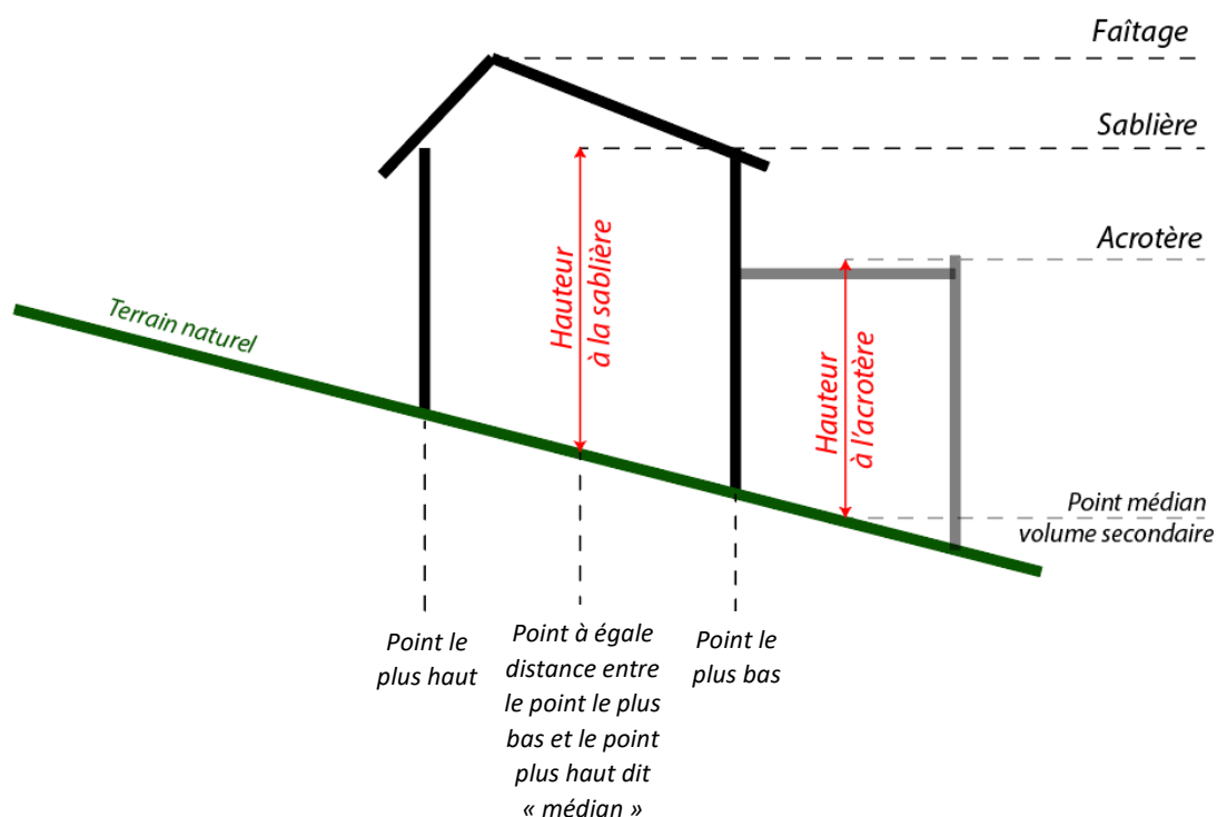
Hauteur à la sablière, hauteur à l'acrotère
